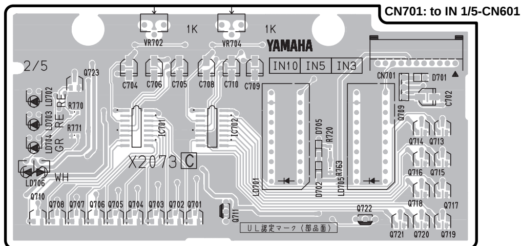
Component side( 部品側 )
