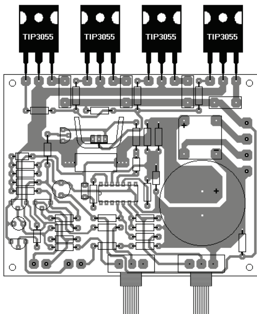
PCB - Transparencia
